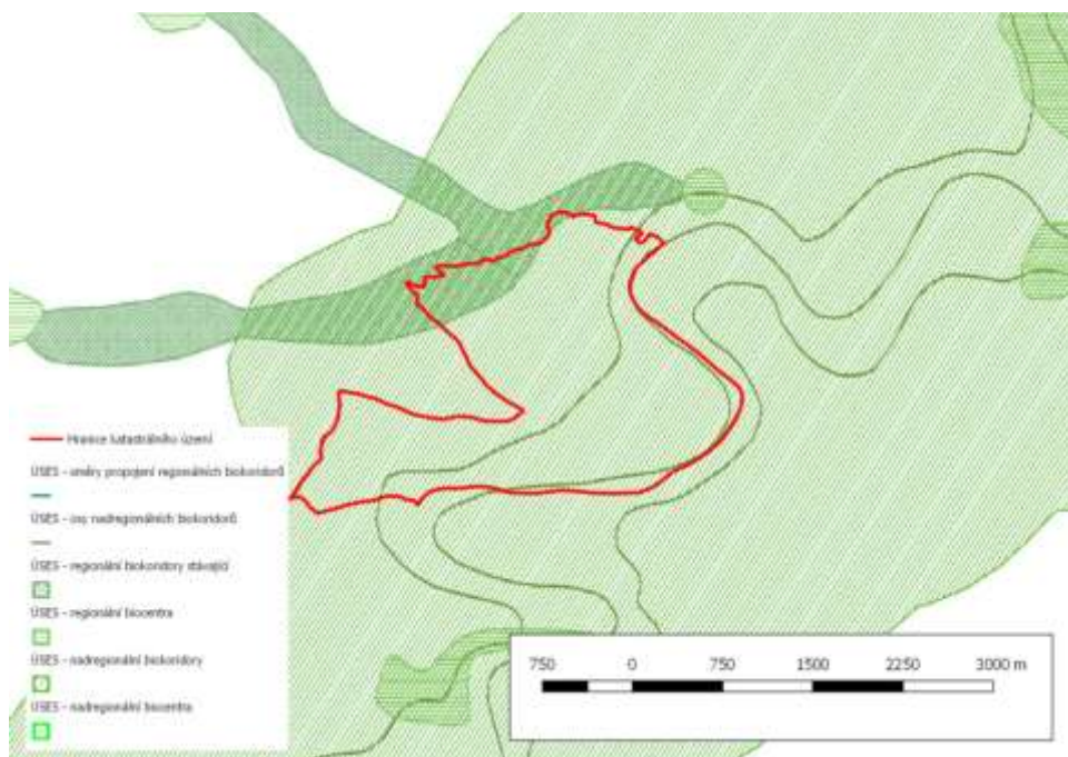
Obrázek 5: Regionální biokoridory
