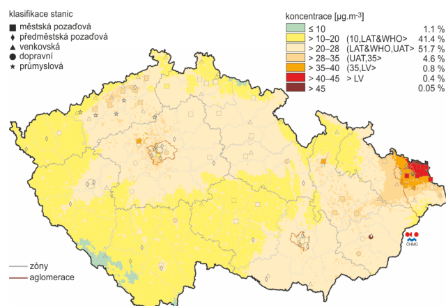
Obr. IV.1.2 Pole roční průměrné koncentrace \text{PM}_{10} , 2014
